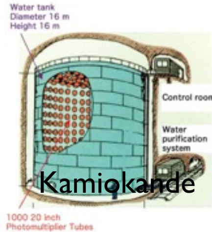
M. Koshiba
